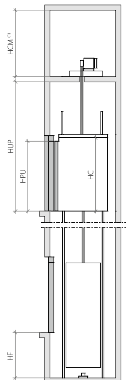
ВЕРТИКАЛЬНЫЙ РАЗРЕЗ
